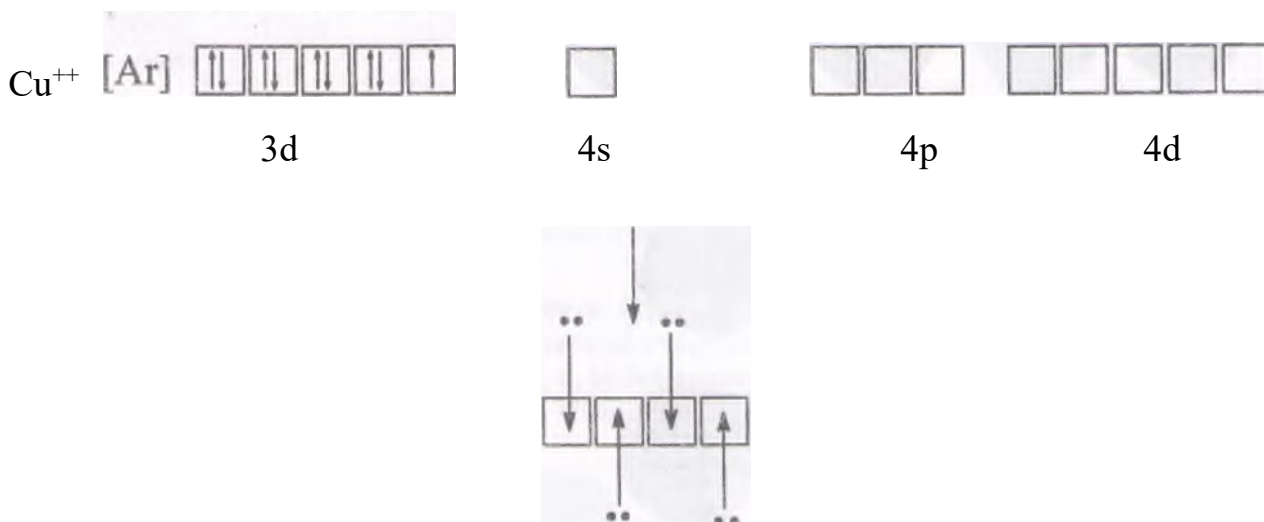
Рис. 4. Образование возможных комплексных связей иона Си за счёт гибридной версии 4s и 4p орбиталов
