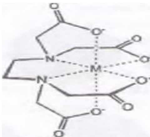
Рис.3. Комплексообразование иона сионами металлов, (M- ион металла)
